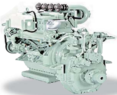
UM4BG1Z [81kW/110PS]
